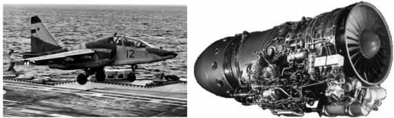
图 5 Su-25TUG 舰载教练攻击机和图曼斯基 R-195 涡喷发动机
